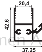
G-2914 ÇEKME PROFİLİ 0,943 kg/m
