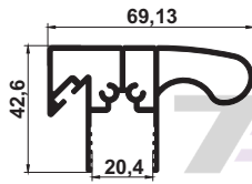
G-2917 TUTAMAKLI ÇEKME 1,266 kg/m
