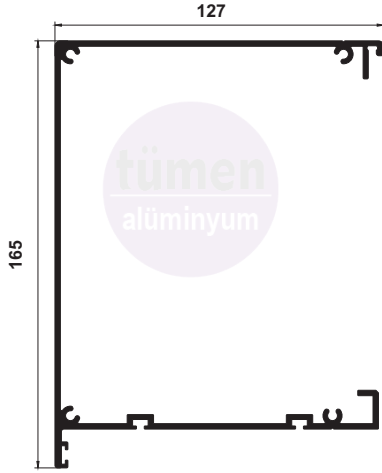
G-2924 MOTOR ŞASE 2,946 kg/m
