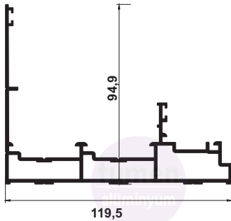
G-2922 YAN KASA 2,1 kg/m
