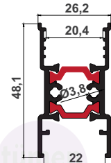
ISI-G-354 YATAY BAZA 0,642 kg/m
