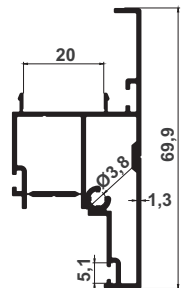
ISI-G-362 VAŞISTAS BAZA 0,851 kg/m
