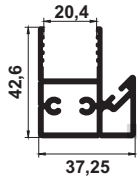
G-2914 ÇEKME PROFİLİ 0,943 kg/m
