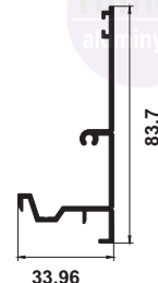
G-2913 KASA DIŞ KAPAK 0,686 kg/m
