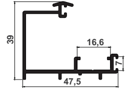
ISI-G-360 YAN KASA ÇITA 0,578 kg/m
