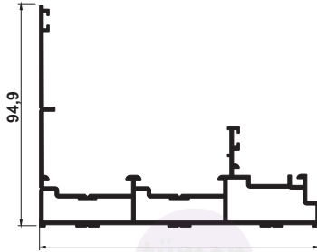
G-2922 YAN KASA 2,1 kg/m
