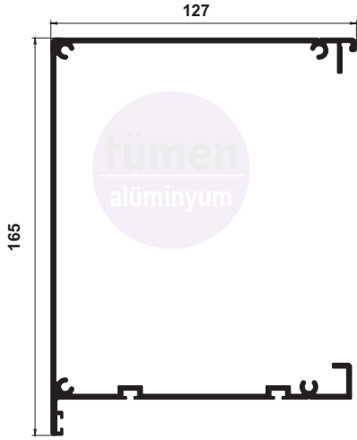
G-2924 MOTOR ŞASE 2,946 kg/m
