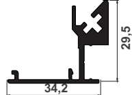
ISI-G-348 ÇEKME BAZA 0,481 kg/m
